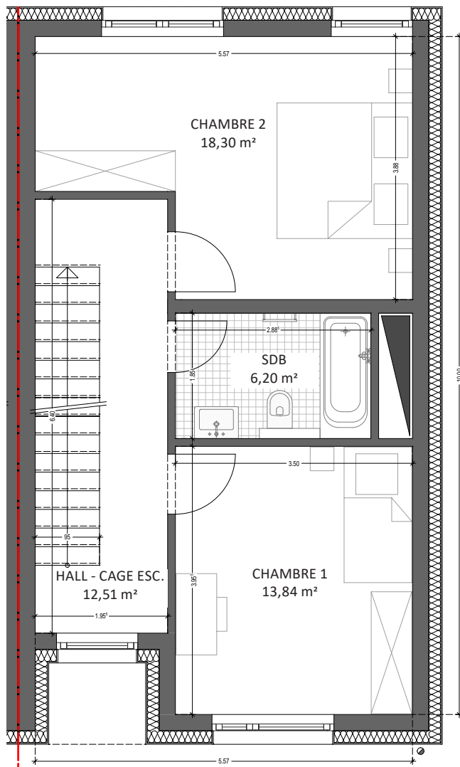
Étage 1
