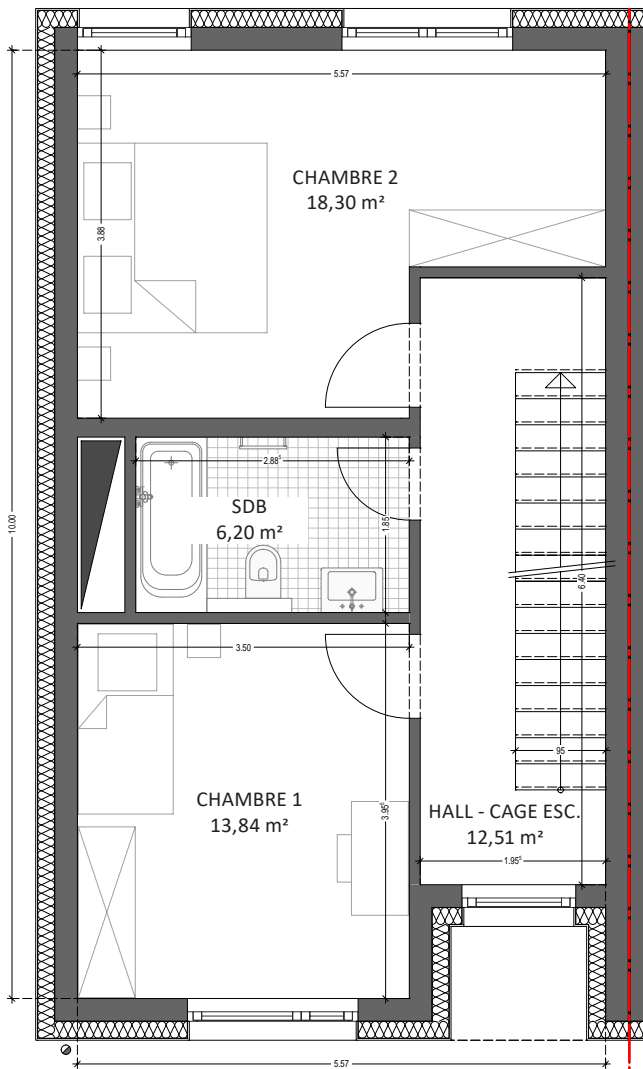
Étage 1
