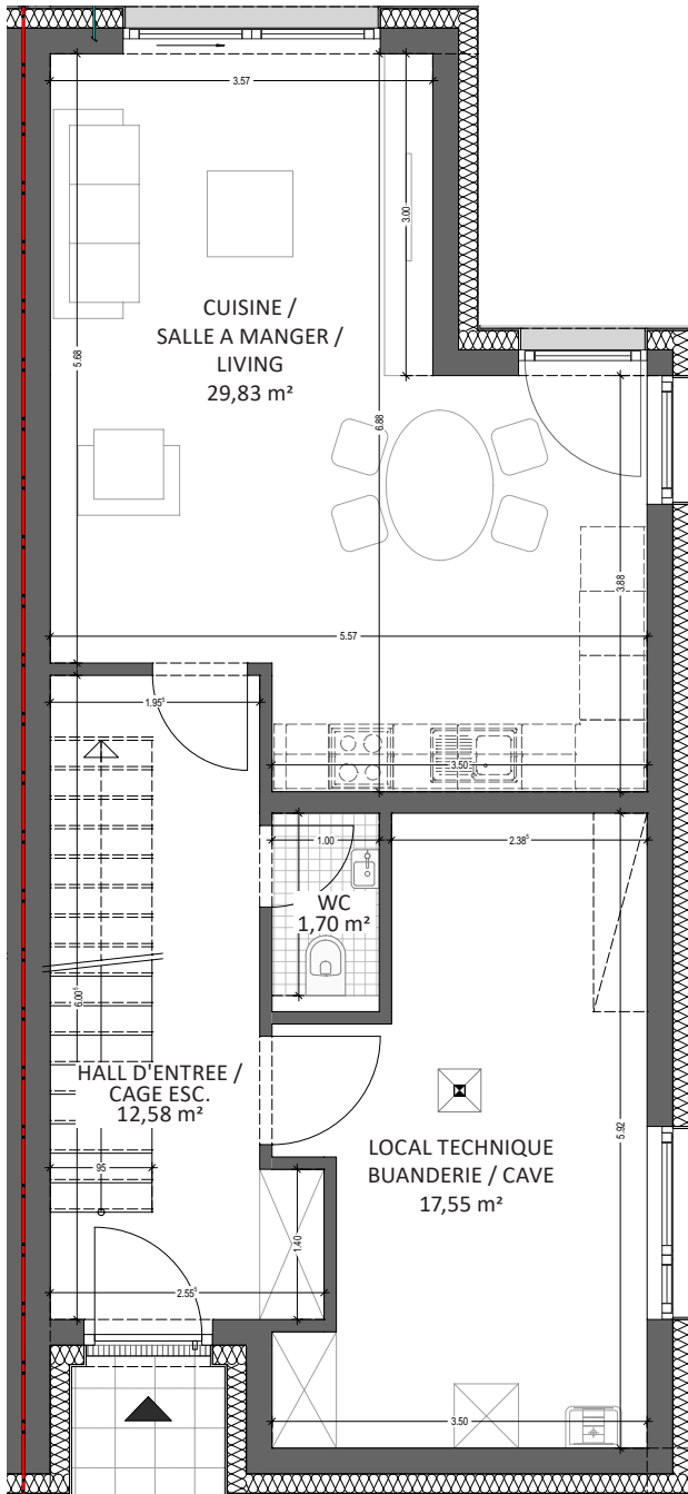
Rez-de-chaussée
