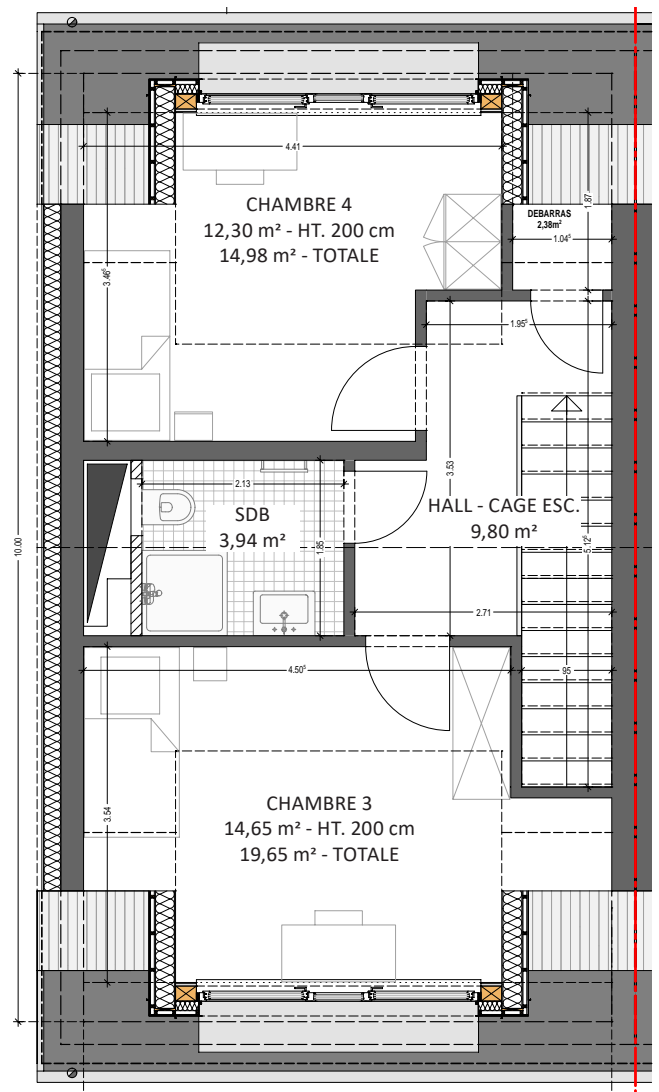
Étage 2
