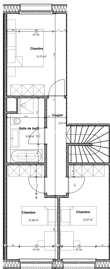
Etage 1
