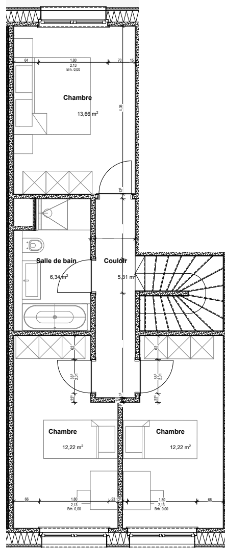
Etage 1
